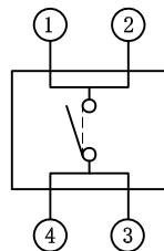
电路图：常开式(N.O) 1个电路1个接点 端子排列（自A方向看）
